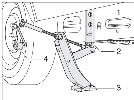
Bild 175 AL-KO-Wagenheber
