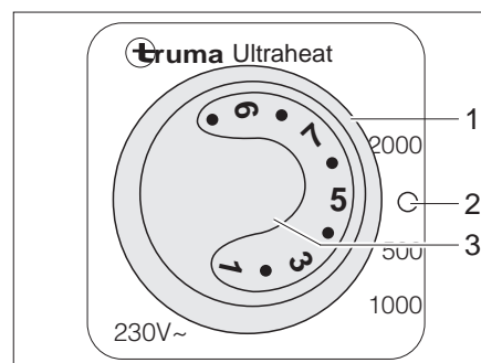
Bild 113 Bedienteil Elektro-Zusatzheizung Ultraheat
