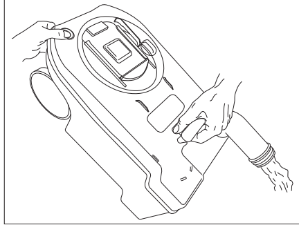
Bild 156 Thetford-Kassette entleeren
