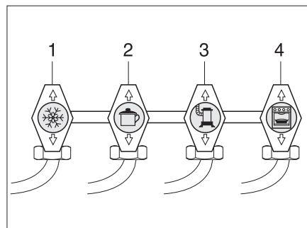
Bild 100 Symbole der Gasabsperrentile
