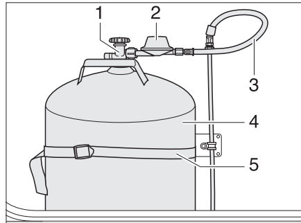
Bild 80 Gaskasten
